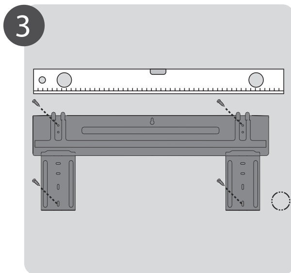
Fije la placa de montaje (Page 11)
