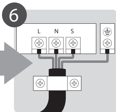
Conexión eléctrica (Page 14)
